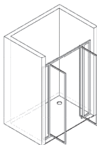
Ușă de duș atipică fără profil în partea de jos (pentru persoanele cu dizabilități)
