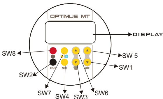
Fig 1. Panoul de comandă pentru OPTIMUS MT
