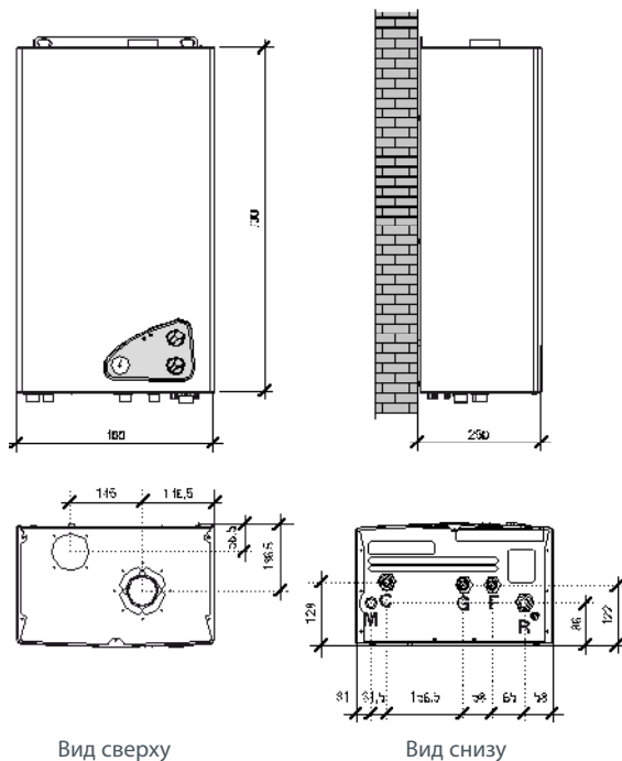
Вид сверху
