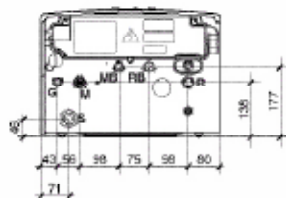
Вид снизу
