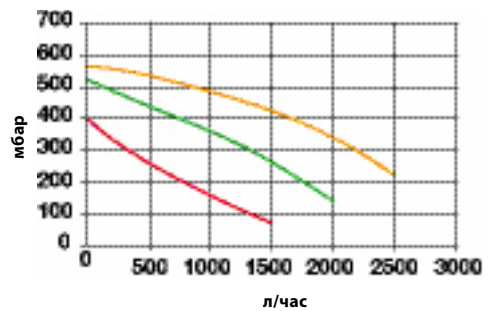
мод. RVA - высокотемпературный контур
