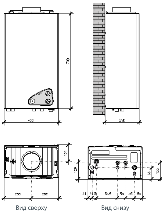
Вид сверху
