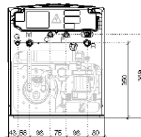
Вид снизу
