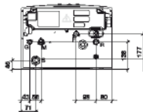
Вид снизу
