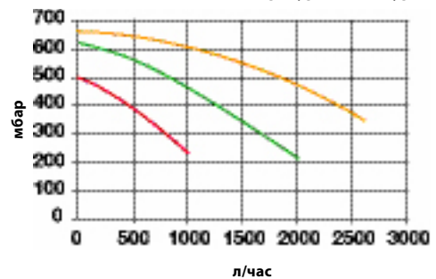
мод. RVA - низкотемпературный контур
