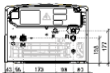
Вид снизу
